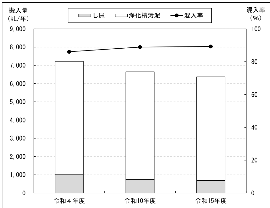
図3-37 し尿及び浄化槽汚泥の搬入量の予測（長島町）
