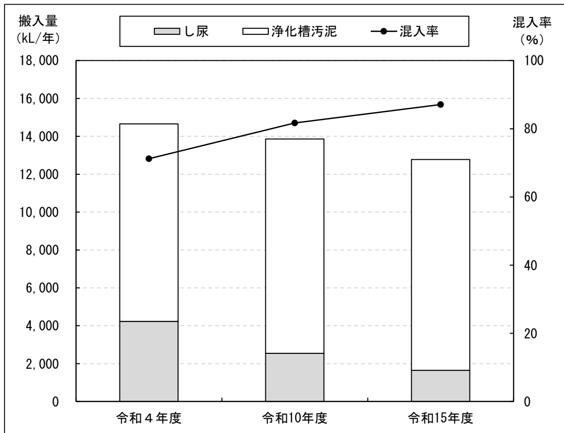
図3-35 し尿及び浄化槽汚泥の搬入量の予測（阿久根市）
