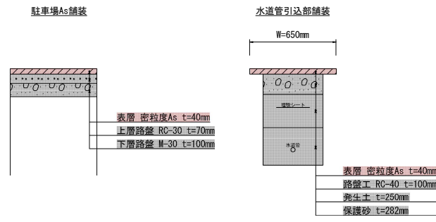
舗装構成図 S=1:20
