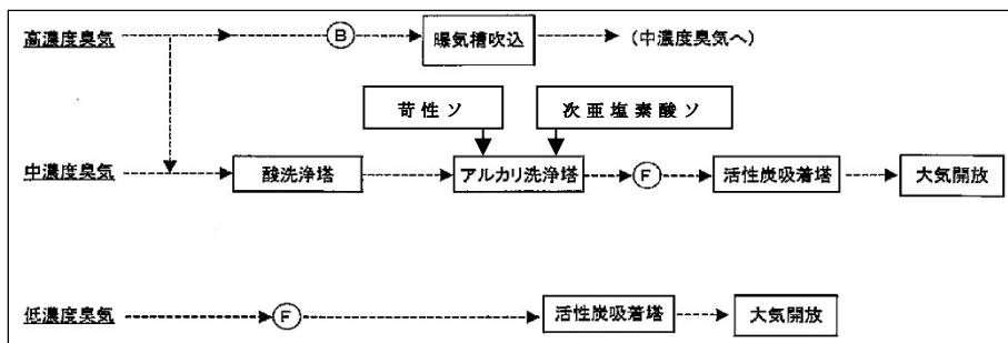
(脱臭処理工程図)
