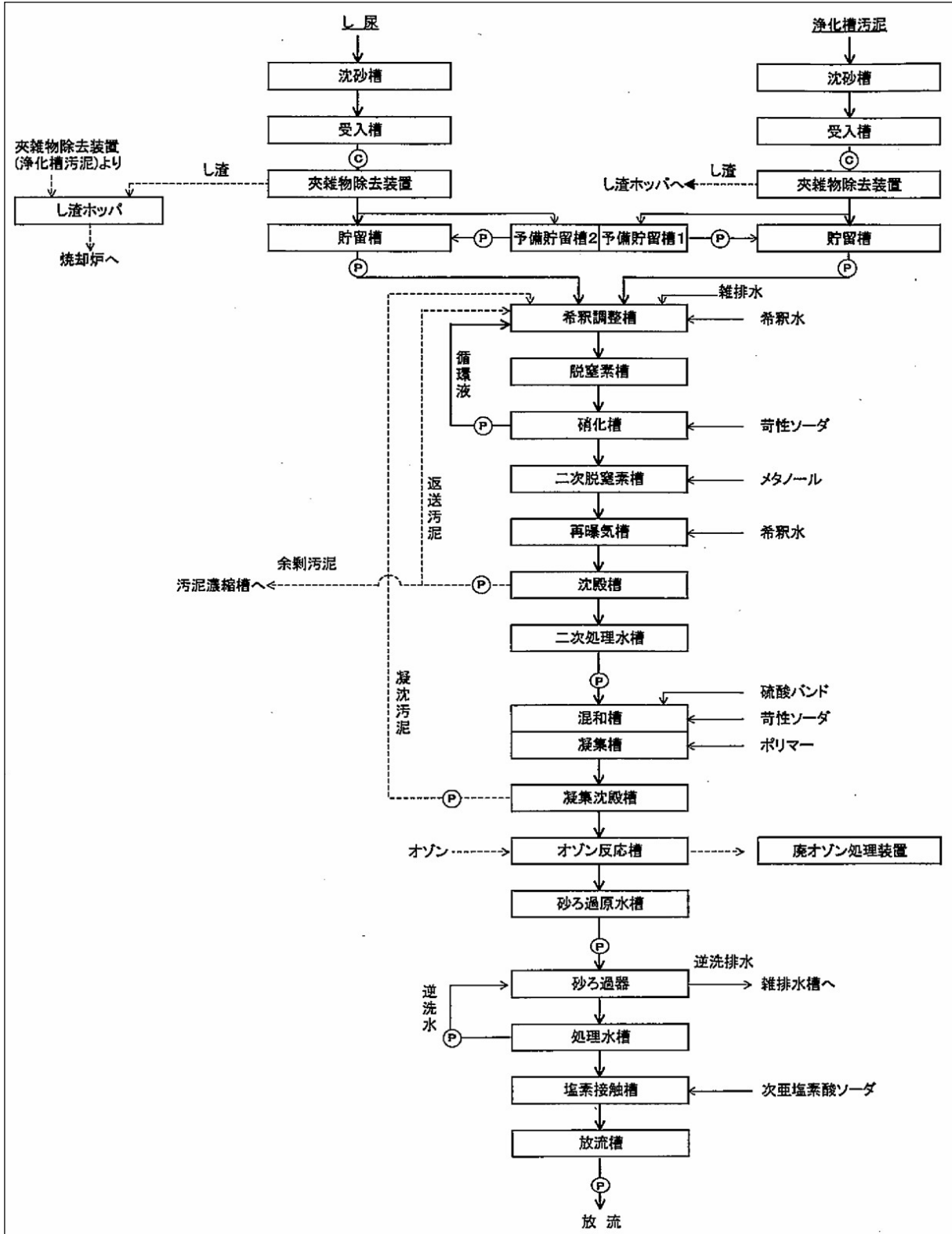
(し尿等処理工程図)
