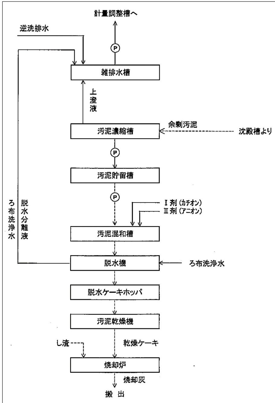
(汚泥処理工程図)
