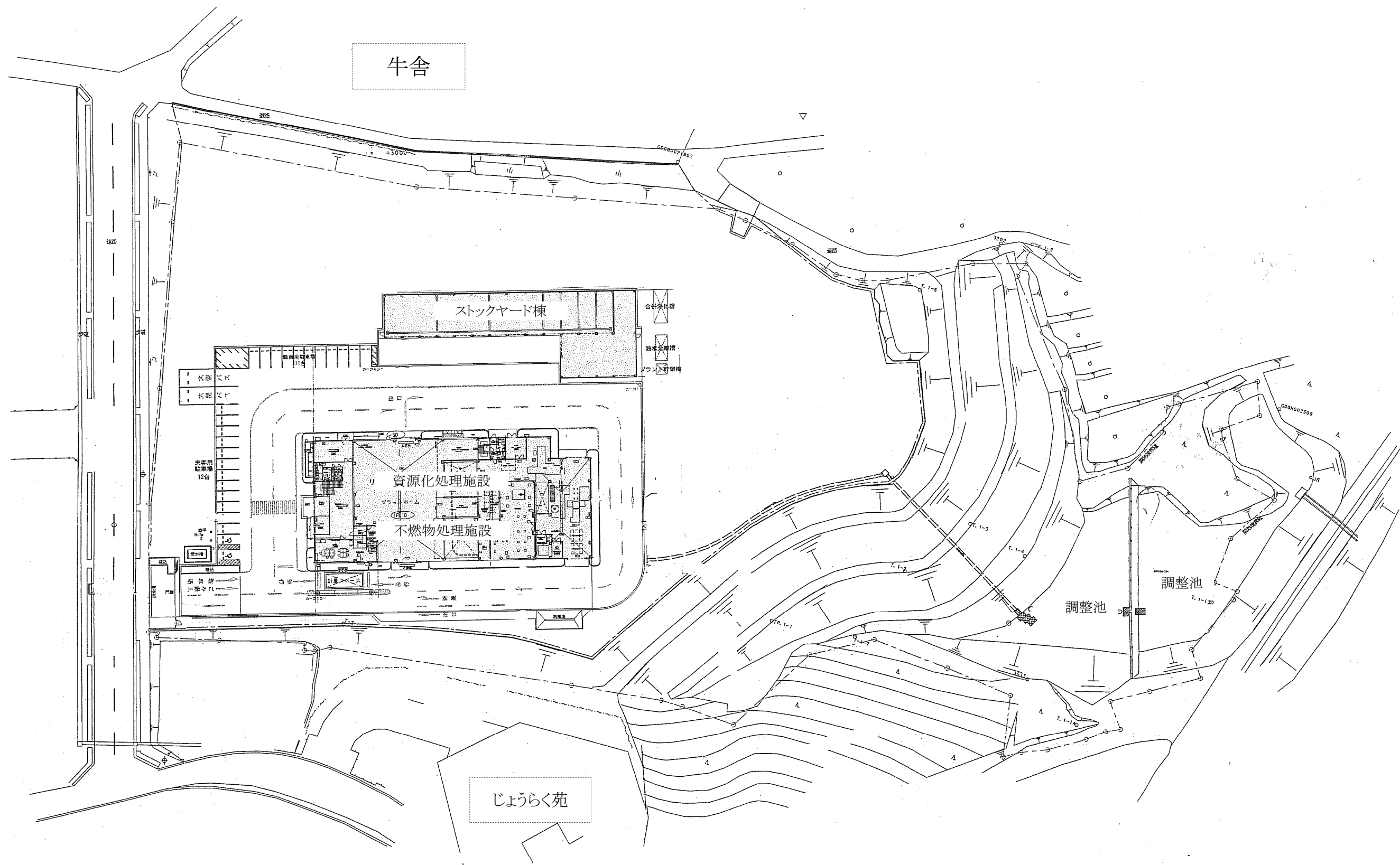
リサイクルセンター 敷地平面図
